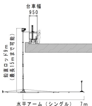
橋梁点検支援ロボット (スタンダードタイプ)
